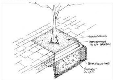
Isometrie (o.M.)
