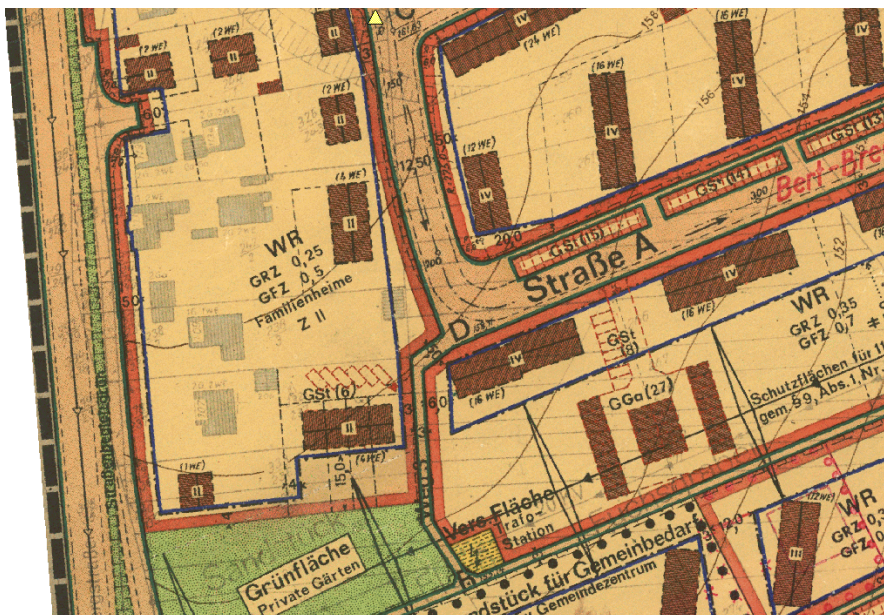
Ausschnitt aus dem Bebauungsplan
