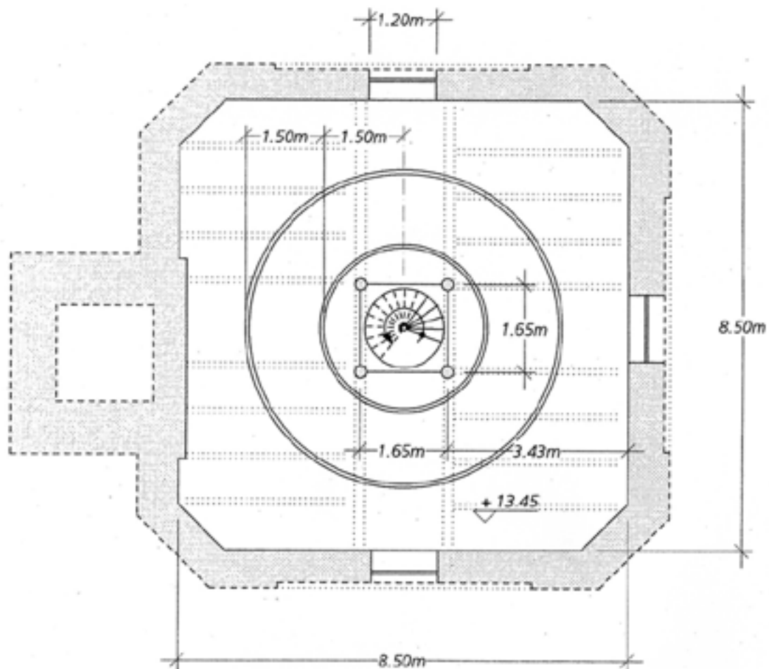
Schlachthofturm □ Grundriss 3. OG
