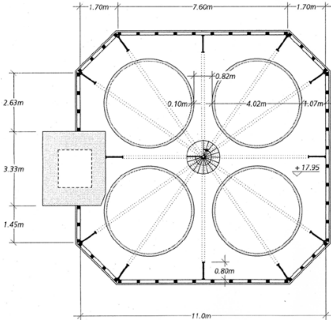
Schlachthofturm □ Grundriss 4. OG
