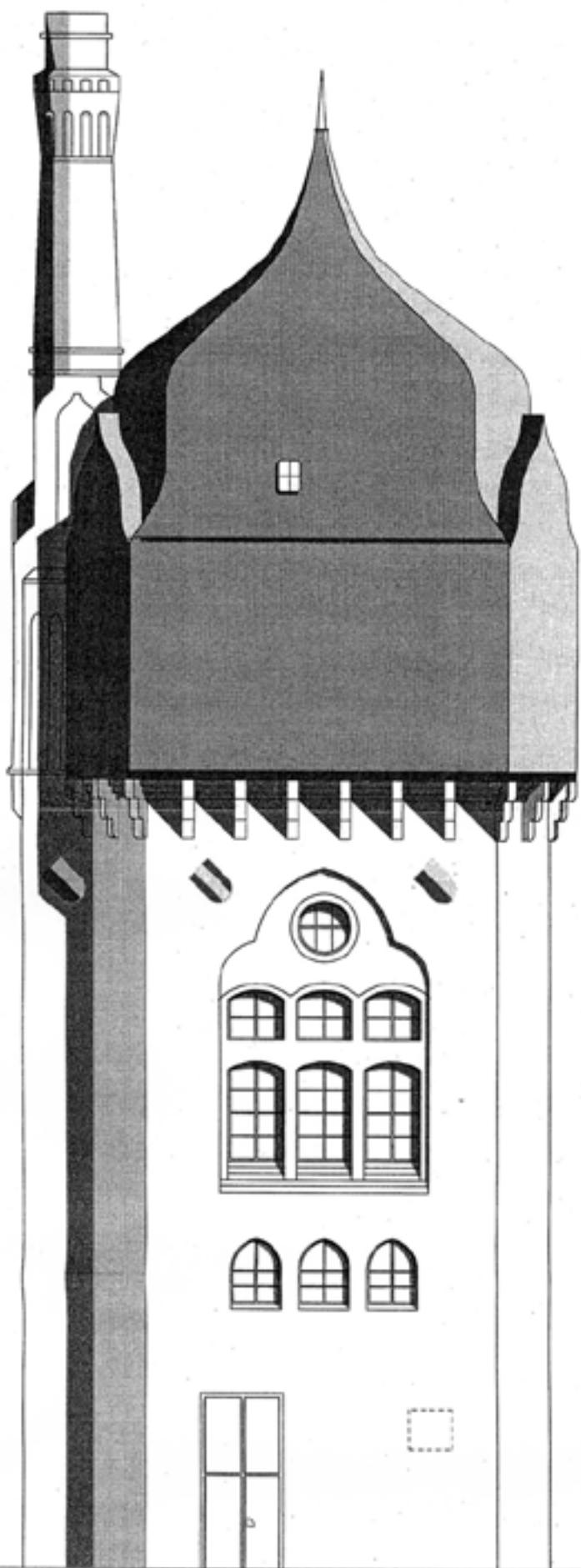
Schlachthofturm, Ansicht Süd
