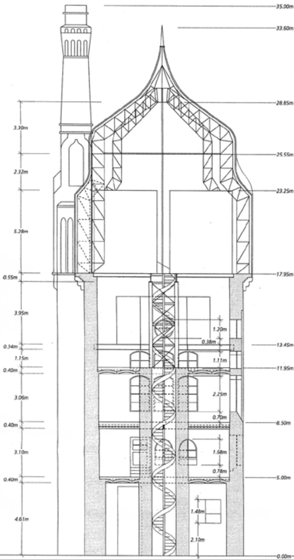
Schlachthofturm, Schnitt West/Ost
