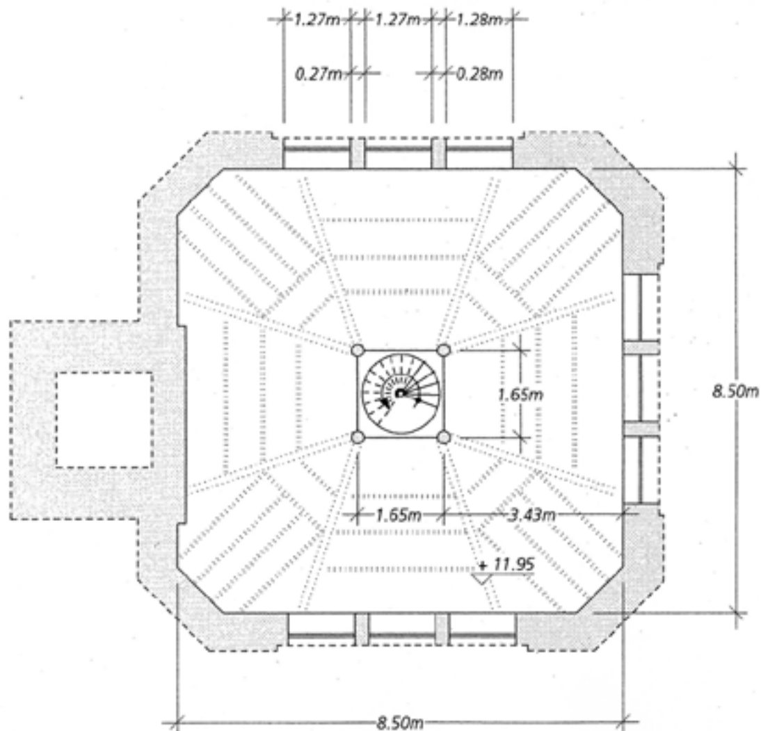
Schlachthofturm □ Grundriss ZG
