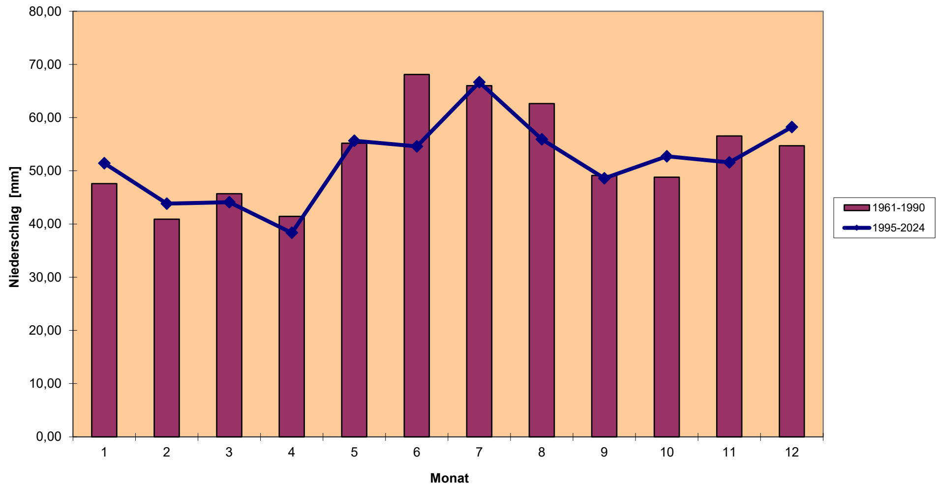
Vergleich der Niederschlagsmessreihen 1961-1990 und 1995-2024 Station Wi-Süd
