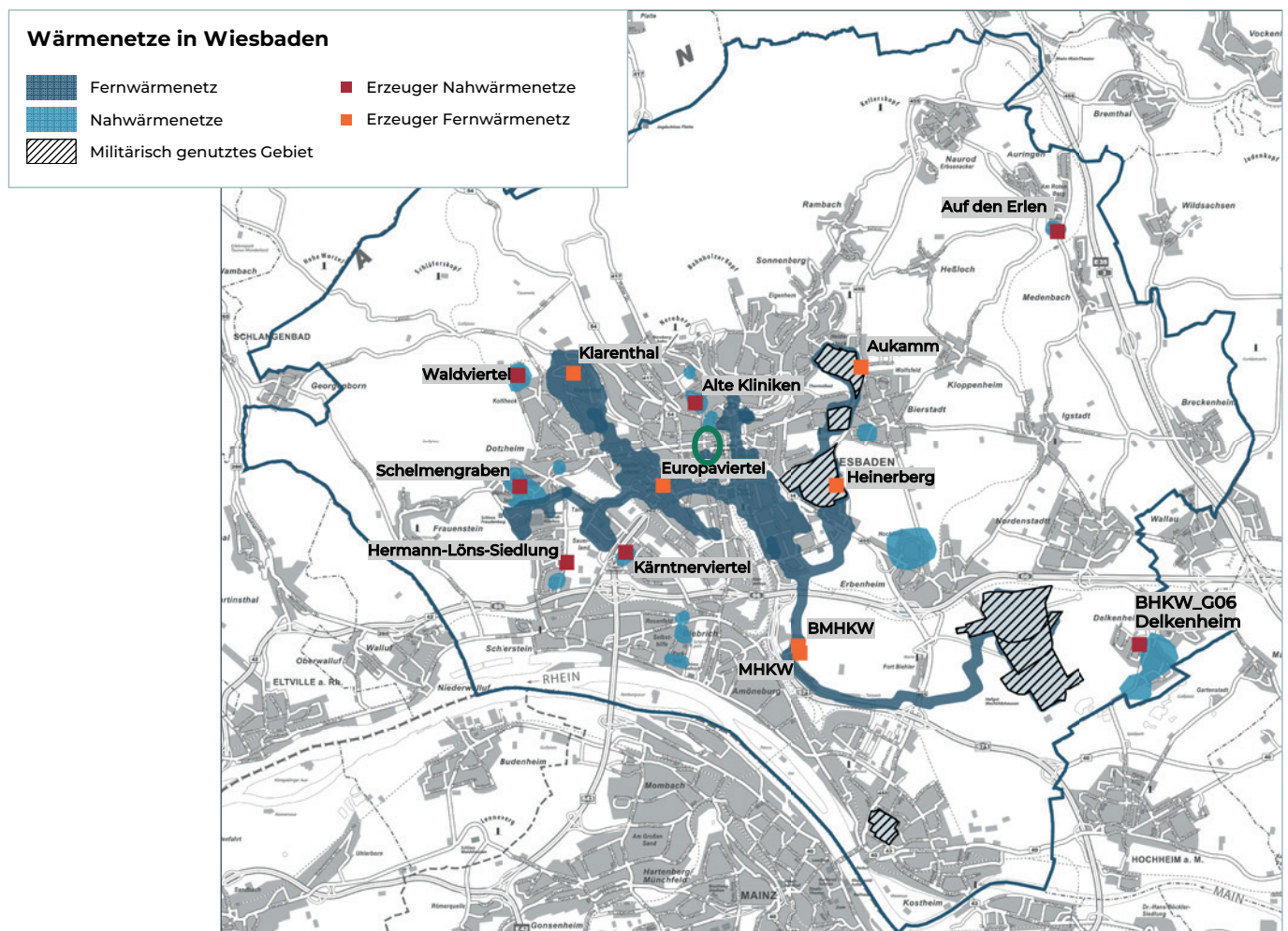
Abbildung 3-16: Wärmeerzeuger und -speicher im Untersuchungsgebiet. Die Grüne Ellipse kennzeichnet das Thermalwärmenetz Schützenhofquelle
