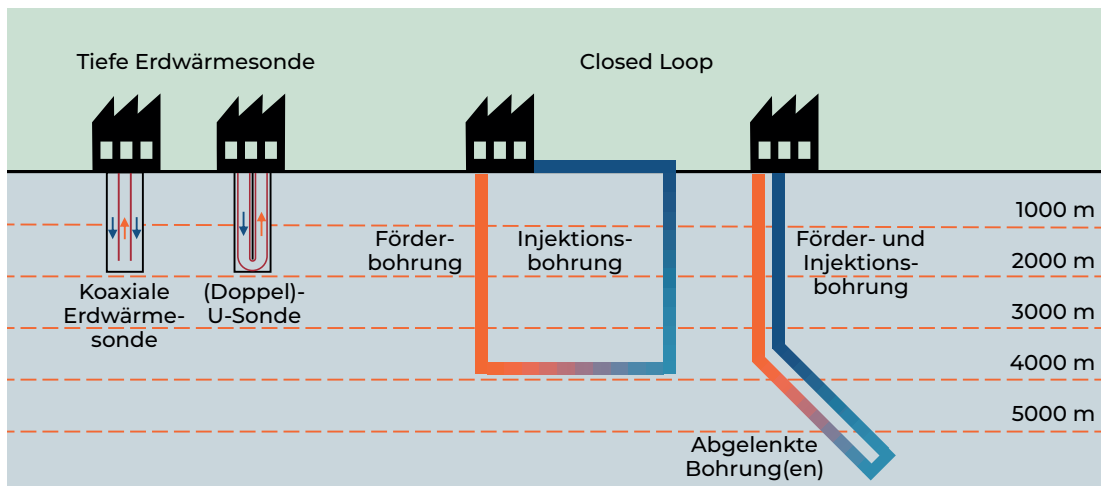
Abbildung 4-12: Schematische Darstellung geschlossener tiefegeothermischer Anlagen (Darstellung Ramboll)
