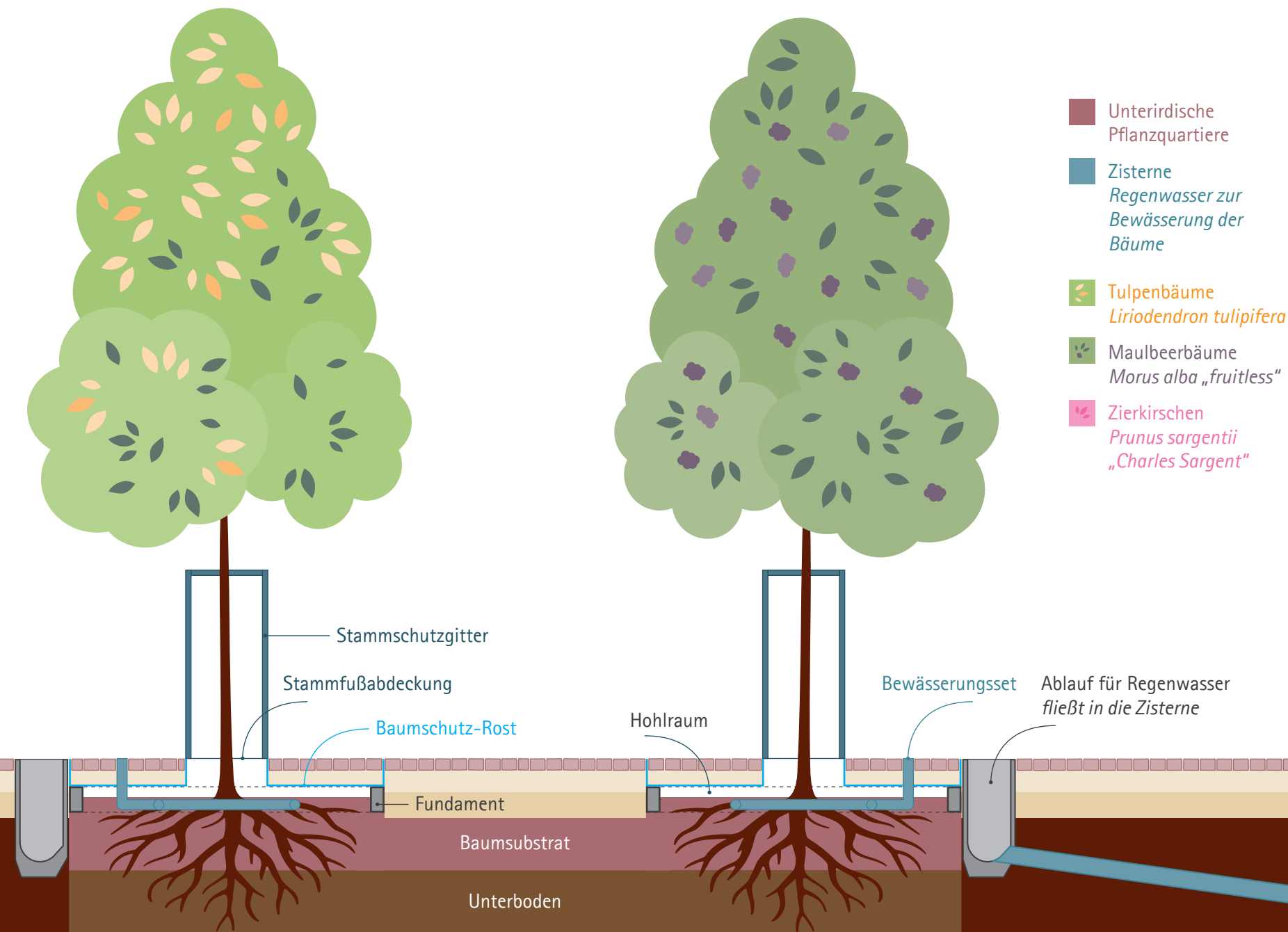
Schnitt A-A
